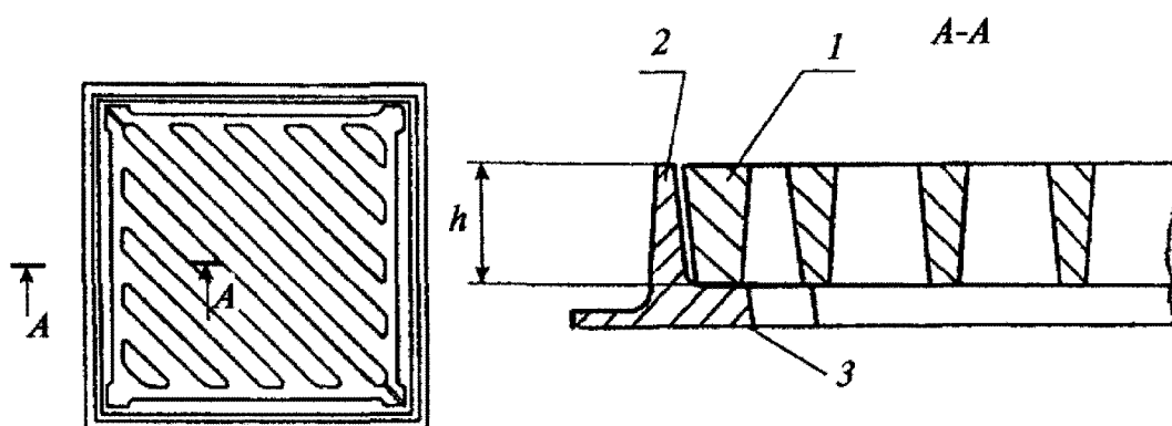
Рисунок Б.1. Дождеприемник ливнесточного колодца
