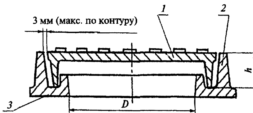
Рисунок А.1. Люк общего назначения
